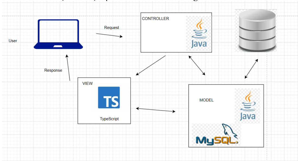
Hình 0: Kiến trúc tổng Thể của hệ thống
